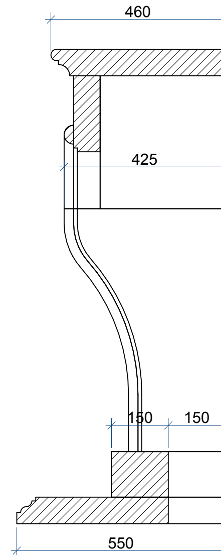
Сечение 2-2
