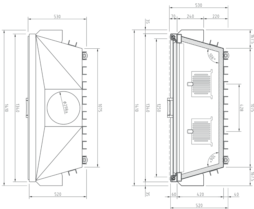
Изображение сверху М 1:10
