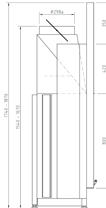
Боковое изображение М 1:20
