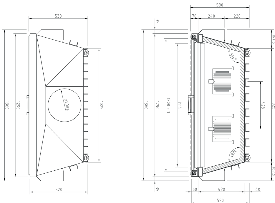
Изображение сверху М 1:10
