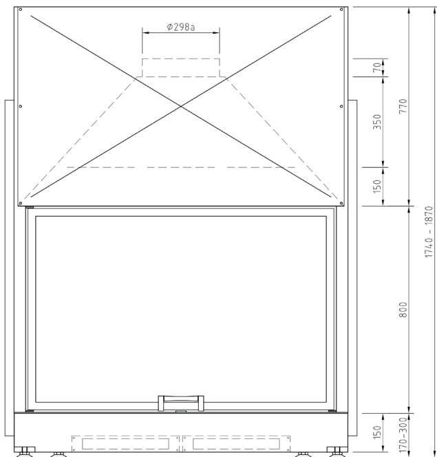
Изображение фронт М 1:20
