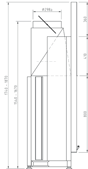
Боковое изображение М 1:20
