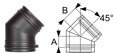
Отвод 45° 7б
