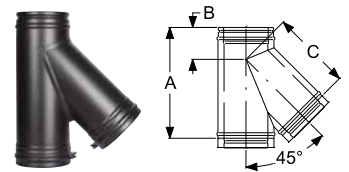
Тройник 45° 6б
