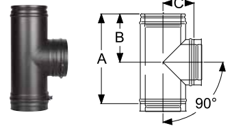
Тройник 90° 6а
