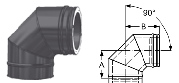
Отвод 90° (Т450 NI) 7а
