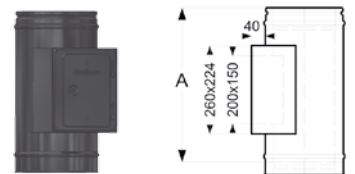
Тройник прочистки для твердого топлива 6с
